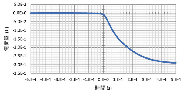
(b) 高压ケーブル内接地線電流の数値積分
