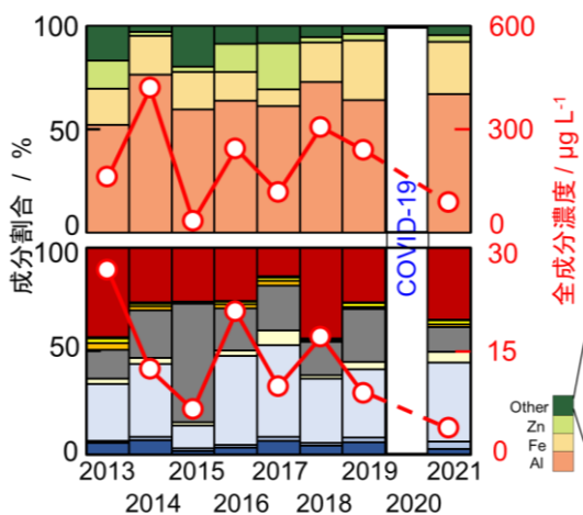
図 3. 富士山頂における雲水中微量金属元素の経年変化
