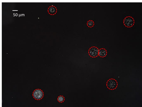
図4 液滴径や硫酸塩濃度の異なる雲滴
