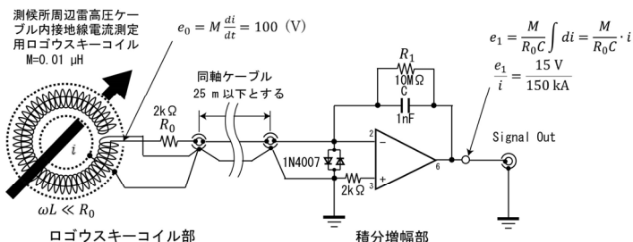
(a) 直撃雷電流測定用ログウスキーコイル電流計基本回路
