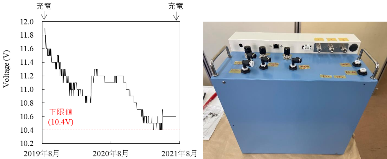
図1. 2019-2021年のCO 2 濃度観測システムのバッテリー電圧値, 写真1. 2021年に導入した新たなCO 2 濃度検出部
