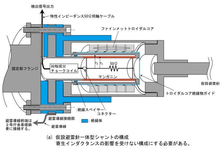
図8 ログウスキーコイルによる避雷針電流一括測定方法
