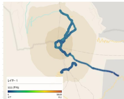
図 富士山の複数の登山道での濃度マップ
